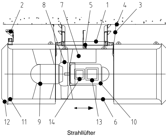
Strahllüfter
